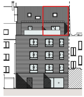
ACHTERGEVEL
